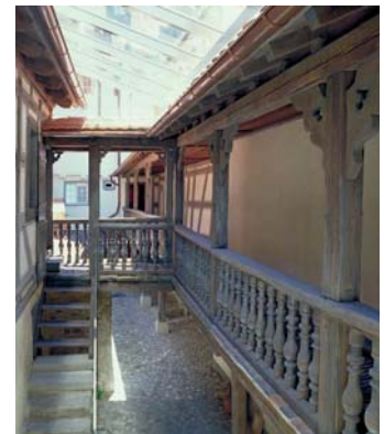
Der Hof erhielt zum Teil eine Glasüberdachung, um die alten Gebäudeteile vor Witterungseinflüssen zu schützen. Foto Maria und Werner Berschneider
